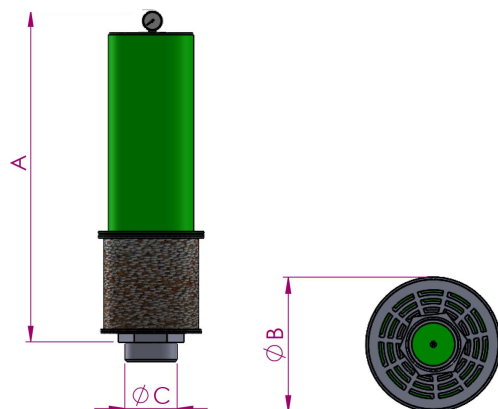
KH-630 A: 695mm B: 222mm C: 4"
